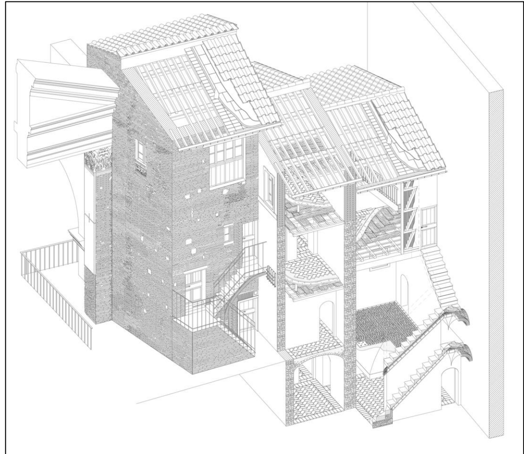
Laboratorio di restauro (prof. F. Geremia). Dettaglio di una nuova scala in legno e spaccato assonometrico di progetto
