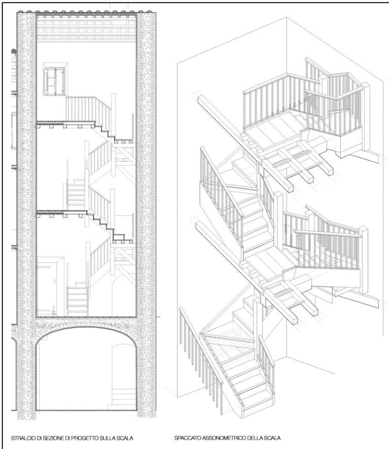
Laboratorio di restauro (prof. F. Geremia). Dettaglio di una nuova scala in legno e spaccato assonometrico di progetto
